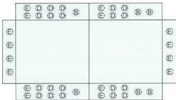
B-12 雙併 600x350x105 B-22 雙併 600x400x105
