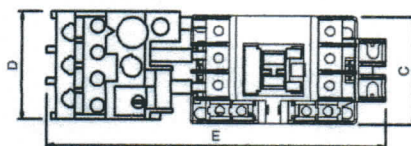
MSO-C-09D~100D 單位：mm
